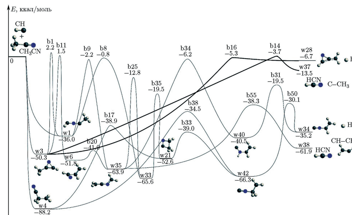
Рисунок 2. Поверхность потенциальной энергии реакции ацетонитрила с метиновым радикалом \text{CH}_3\text{CN} + \text{CH} .
