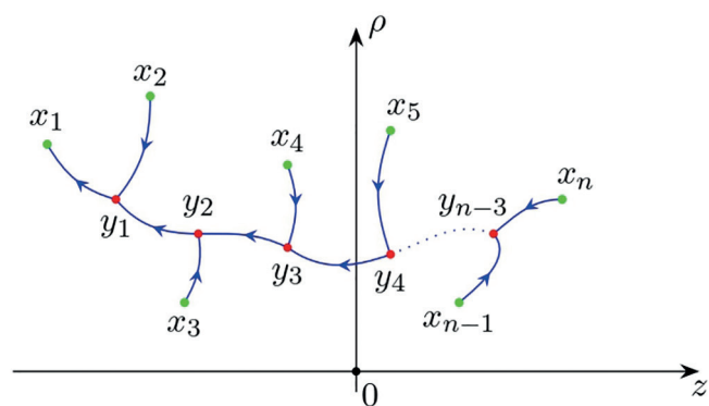
Рисунок 1. Вильсоновский матричный элемент в comb канале в виде графа. Локальные координаты пространства AdS_2 обозначены как \rho и z . Конформная граница пространства соответствует \rho=0
