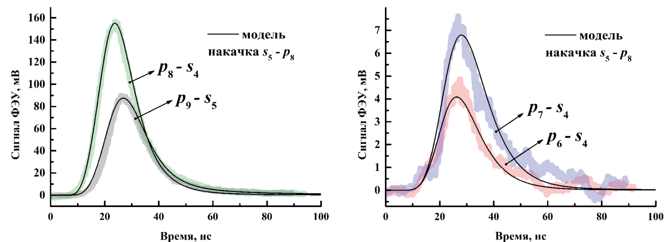
Рисунок 2. Сигналы флуоресценции на переходах между уровнями при давлении в камере P = 300 Торр и температуре газа в зоне разряда T = 400 \pm 10 К
