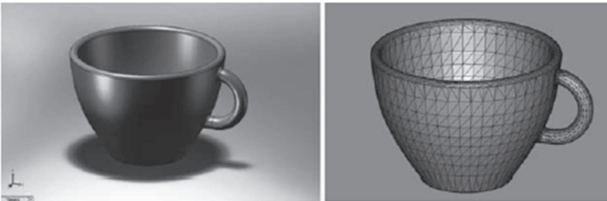
Рис. 2.2. Модель, выполненная в среде САПР (слева) и преобразованная в STL формат (справа)
